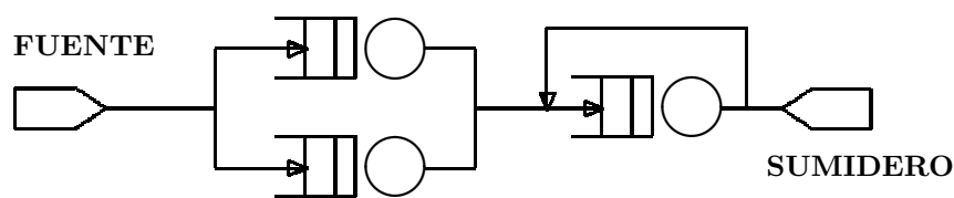
Figura 4.2: Ejemplo de red de colas abierta.
